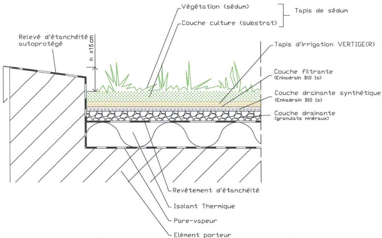
Figure 11 – Coupe type sur relevé (sans zone stérile), élément porteur en maçonnerie, 0\% \leq \text{pente} < 2\%
